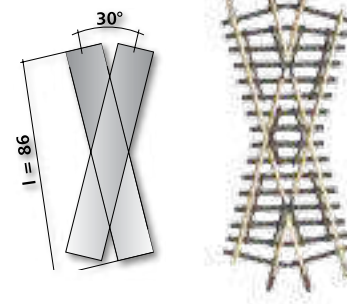
K 2, 30° K 2, 30° Art.-Nr. 83170
