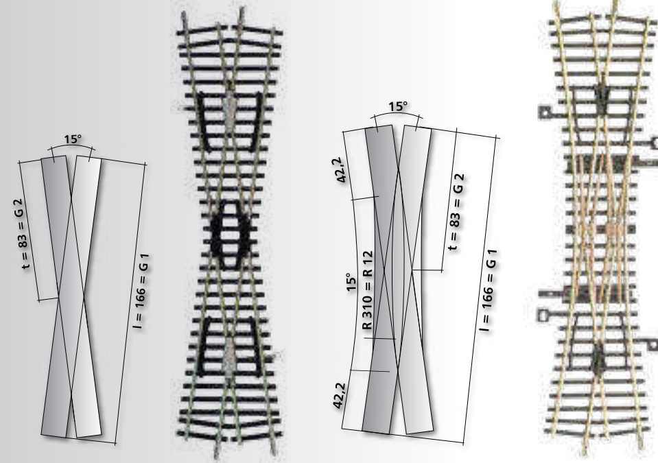
K 1, 15° K 1, 15° Art.-Nr. 83161
