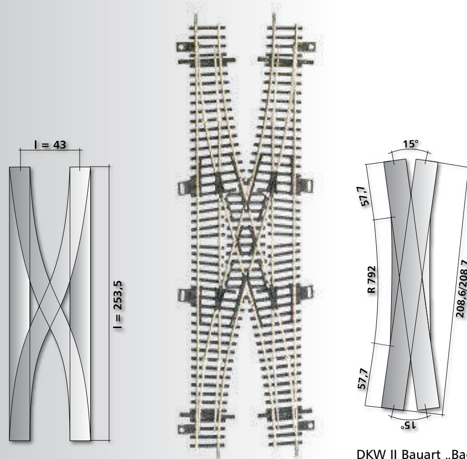
DGV 30° Herzstückwinkel Weichen 15° DGV 30°, frog angle 15° Art.-Nr. 83210
