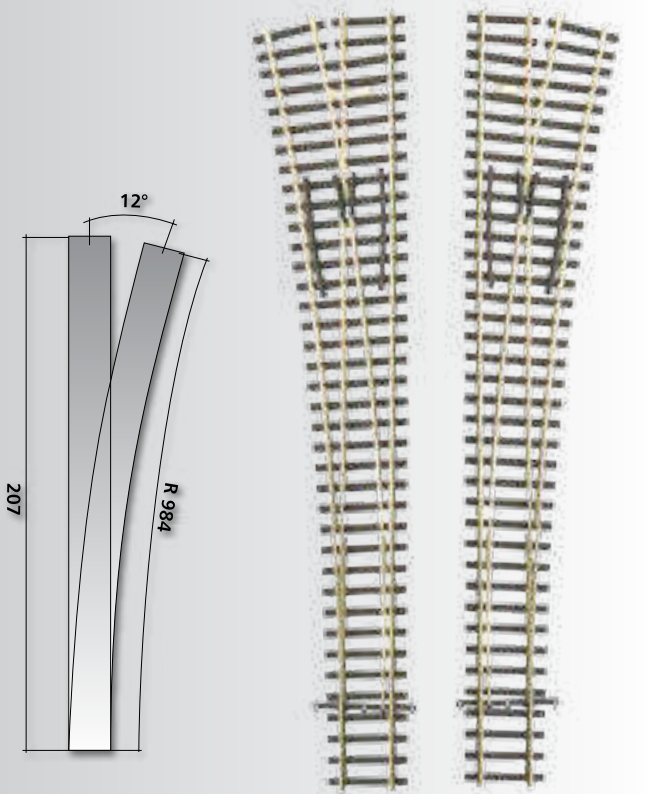
EW 3, links 12°, 207 mm EW 3, left points 12°, 207 mm Art.-Nr: 83342
