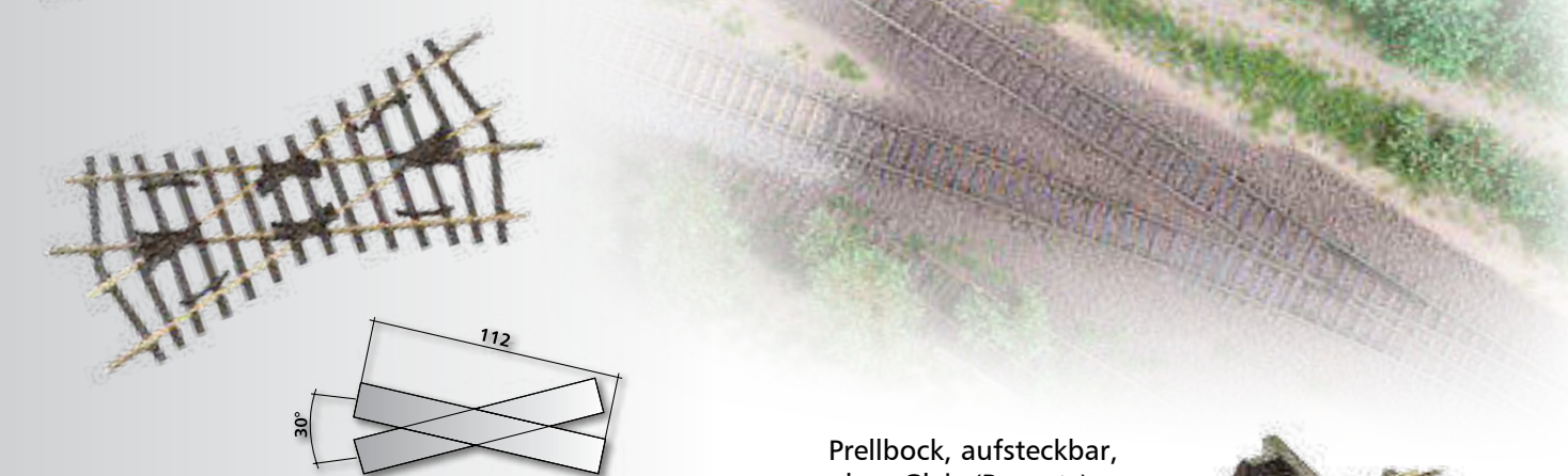
K 30 – Kreuzung 30° K 30 – 30° crossing
