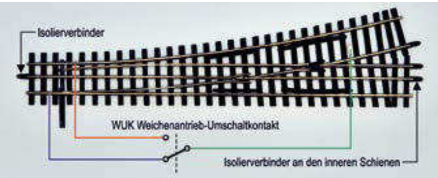
Bei Dreischienenweichen mit Abzweig in H0 sind vier Isolierverbinder anzubringen.
